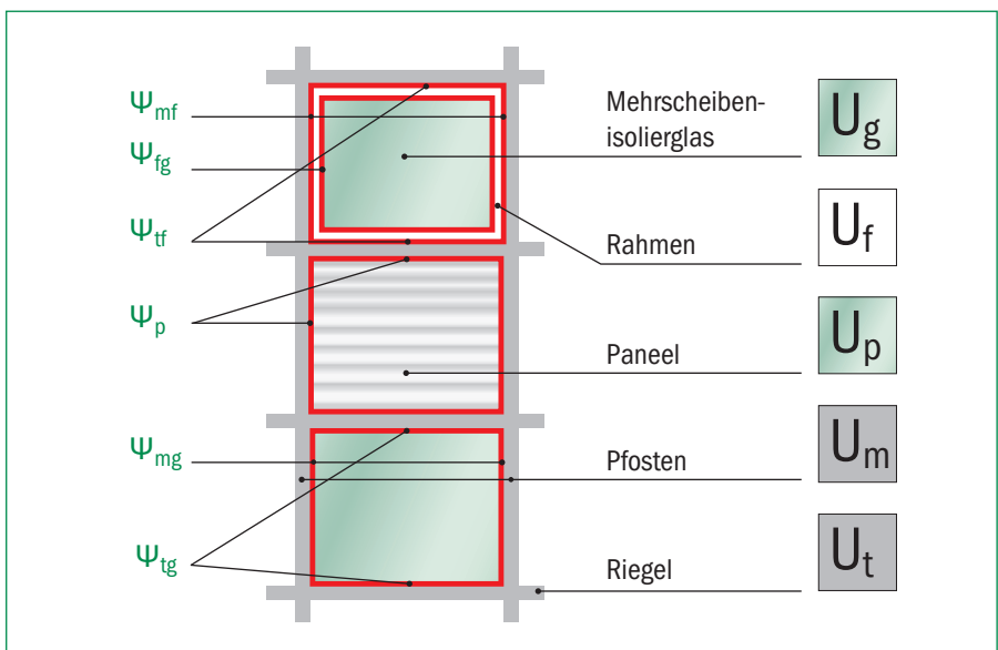
Abb. 13: Musterfassadenelement gemäß EN ISO 12631 [3]
